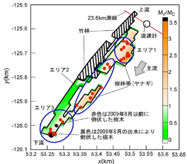
図-3 倒伏力の解析値 M_v/M_c （緑色→茶色に向かうほど大きい）と倒伏した樹木の位置（赤丸）
