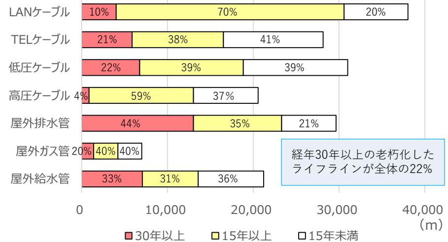
神戸大学のライフライン経年状況 (R6.5.1現在)
